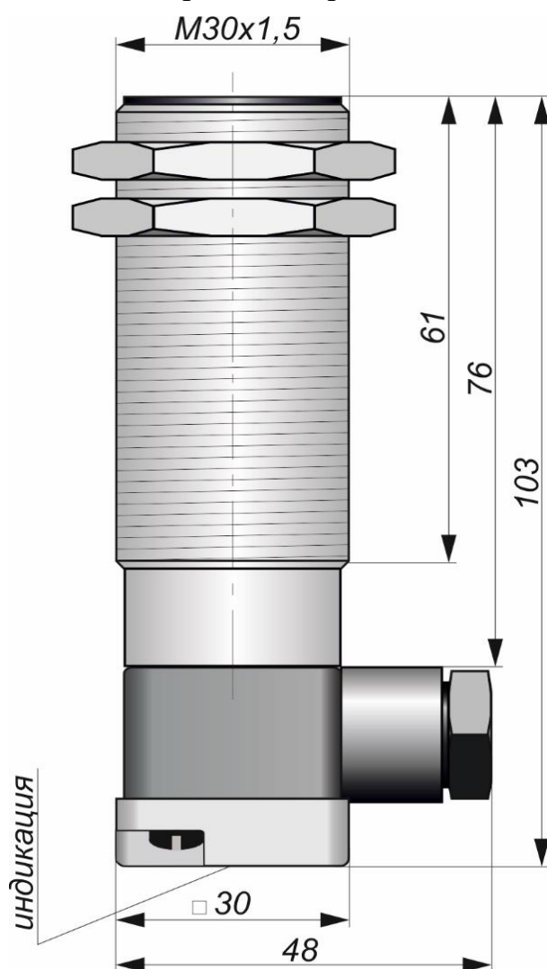
Габаритный чертеж
